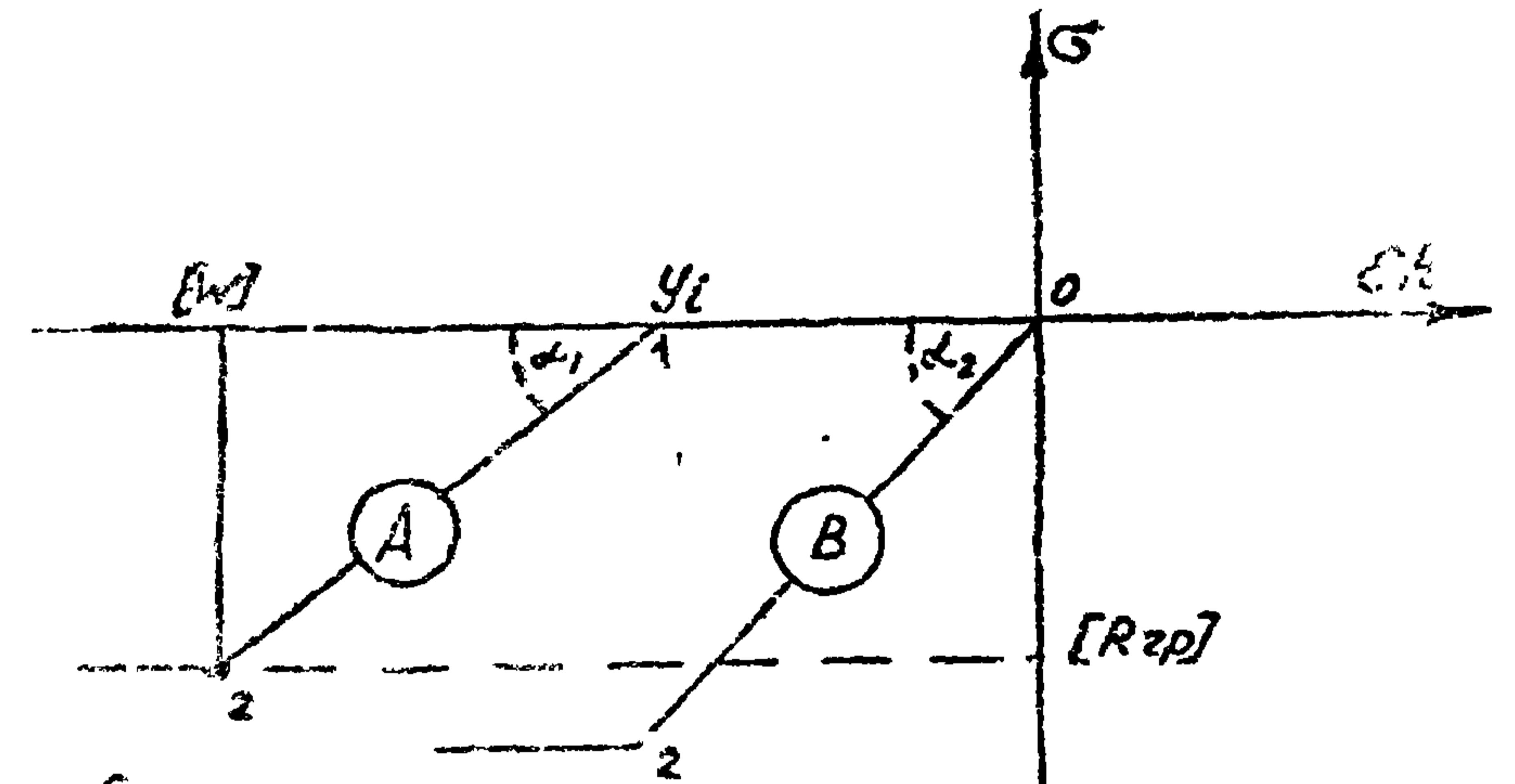
рис. 3 Диаграмма работы стержня модели основания
